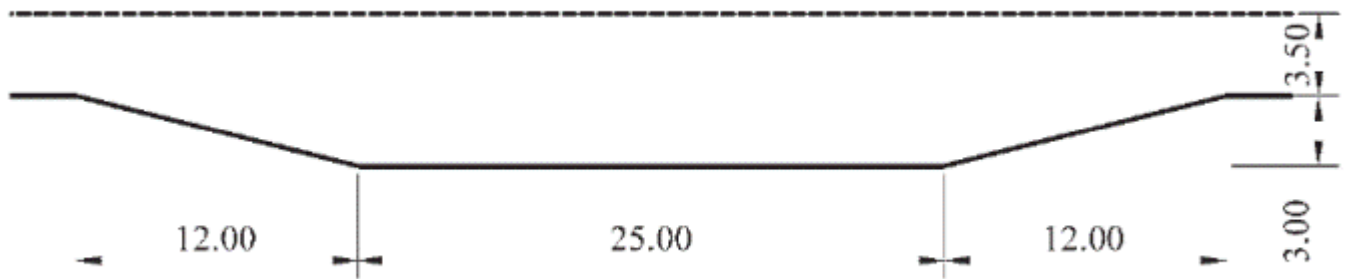
Slika 20. Prostor i oznake prostora za izvođenje poligonske radnje "zaustavljanje vozila na autobuskom stajalištu, radi izlaska i ulaska putnika i polazak sa autobuskog stajališta" (za osposobljavanje kandidata za vozače vozila kategorija D1 i D)
