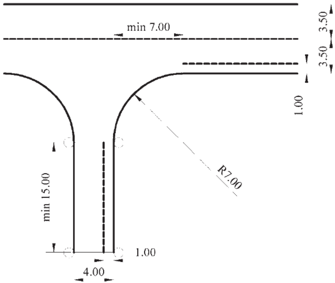
Slika 15. Prostor i oznake prostora za izvođenje poligonske radnje "parkiranje vozila pod pravim uglom, vožnjom unazad, zbog utovara-istovara" (za osposobljavanje kandidata za vozače motornih vozila kategorija C1 i C)
