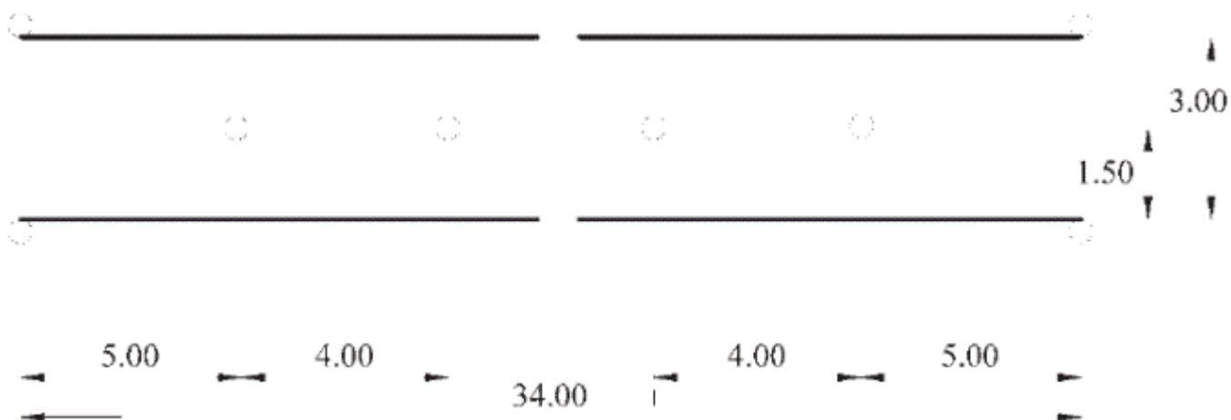
Slika 1. Prostor i oznake prostora za izvođenje poligonske radnje "vožnja po pravcu i zaustavljanje" (za osposobljavanje kandidata za vozače motornih vozila kategorija AM, A1, A2 i A)
