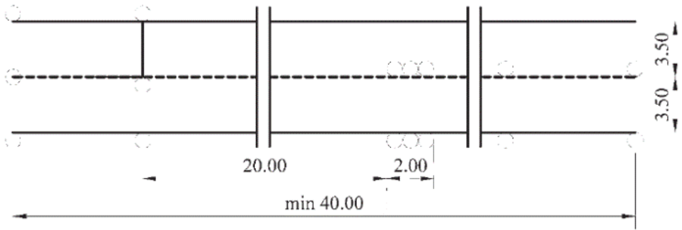
Slika 14. Prostor i oznake prostora za izvođenje poligonske radnje "vožnja napred sa promenom stepena prenosa i unazad sa promenom saobraćajne trake" (za osposobljavanje kandidata za vozače motornih vozila kategorija C1 i C)
