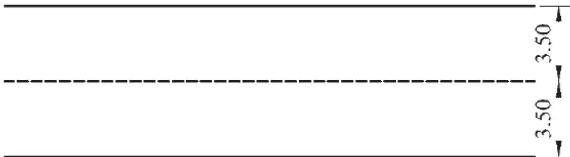
Slika 16. Prostor i oznake prostora za izvođenje poligonske radnje "odvajanje i spajanje vučnog i priključnog vozila" (za osposobljavanje kandidata za vozače vozila kategorija C1E i CE)
