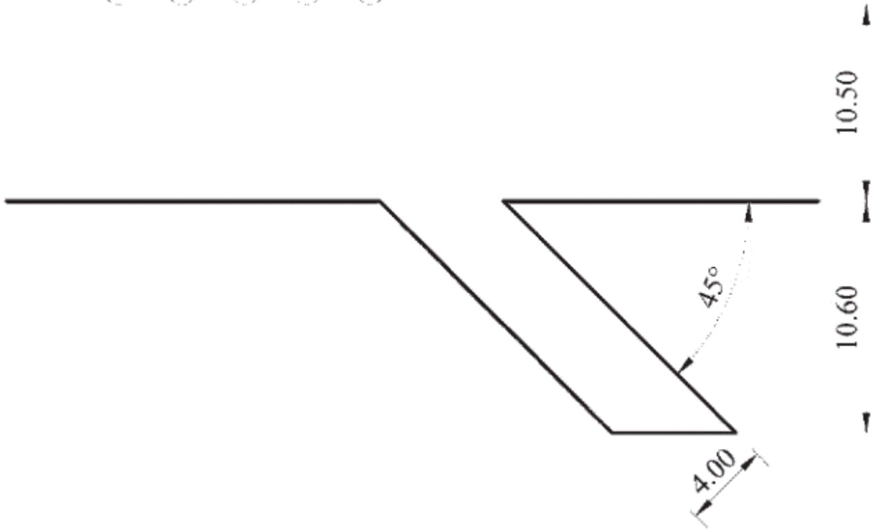
Slika 19. Prostor i oznake prostora za izvođenje poligonske radnje "zaustavljanje vozila na peronu, radi izlaska i ulaska putnika i polazak sa perona" (za osposobljavanje kandidata za vozače vozila kategorija D1 i D)
