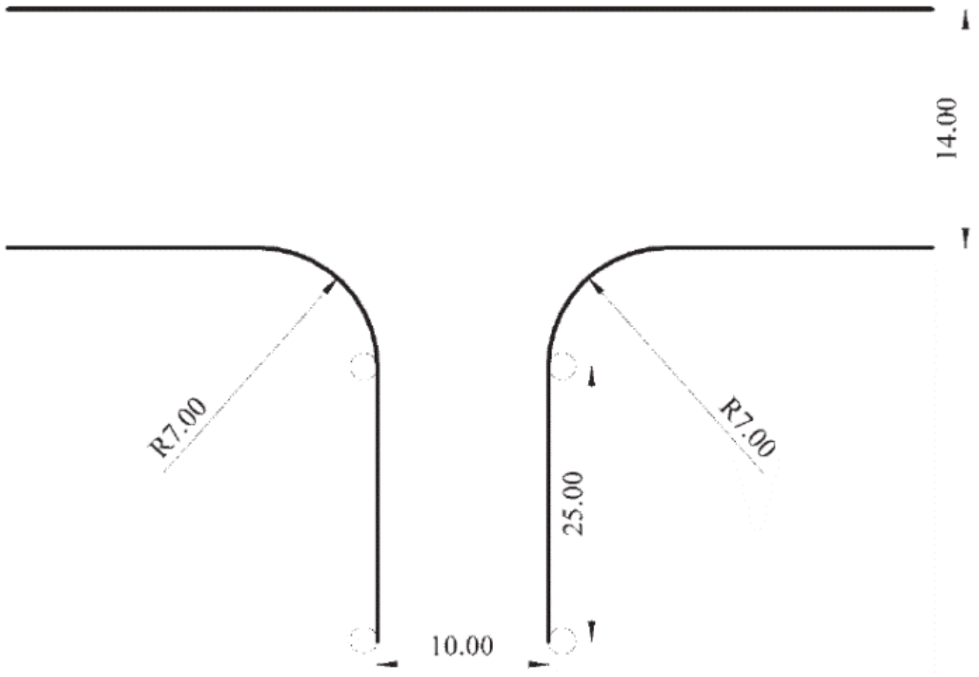
Slika 18. Prostor i oznake prostora za izvođenje poligonske radnje "vožnja unazad sa skretanjem ulevo, odnosno udesno, pod pravim uglom" (za osposobljavanje kandidata za vozače vozila kategorija C1E i CE)
