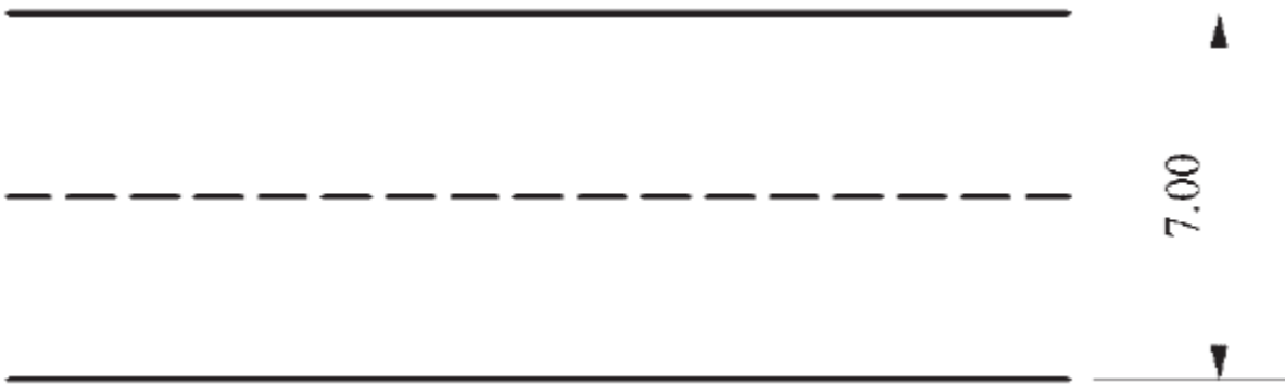
Slika 8. Prostor i oznake prostora za izvođenje poligonske radnje "polukružno okretanje vozila sa najviše tri potpuna manevra na prostoru širine dve saobraćajne trake" (za osposobljavanje kandidata za vozače motornih vozila kategorija B1 i B)
