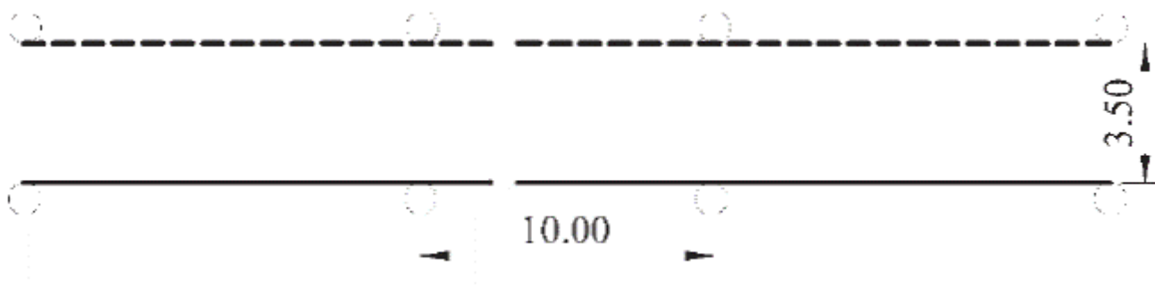
Slika 25. Prostor i oznake prostora za izvođenje poligonske radnje "vožnja napred sa promenom stepena prenosa i unazad u istoj saobraćajnoj traci" (za osposobljavanje kandidata za vozače vozila kategorije F)
