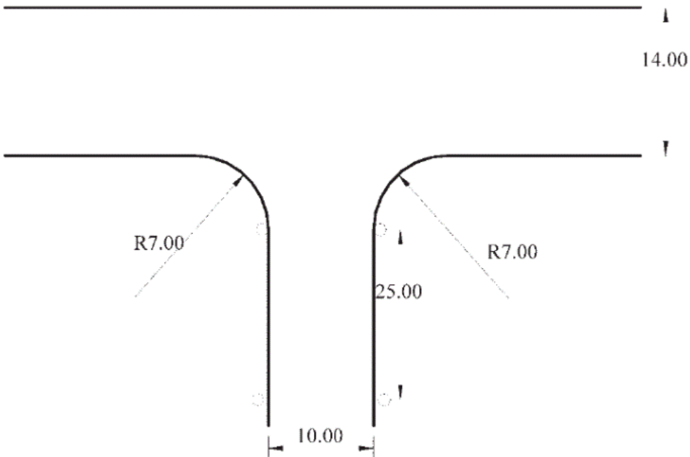
Slika 23. Prostor i oznake prostora za izvođenje poligonske radnje "vožnja unazad sa skretanjem ulevo, odnosno udesno, pod pravim uglom" (za osposobljavanje kandidata za vozače vozila kategorija D1E i DE)
