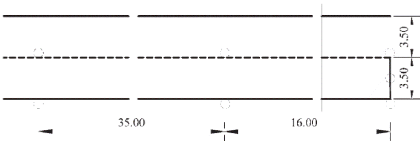
Slika 10. Prostor i oznake prostora za izvođenje poligonske radnje "kočenje i zaustavljanje" (za osposobljavanje kandidata za vozače motornih vozila kategorija B1 i B)
