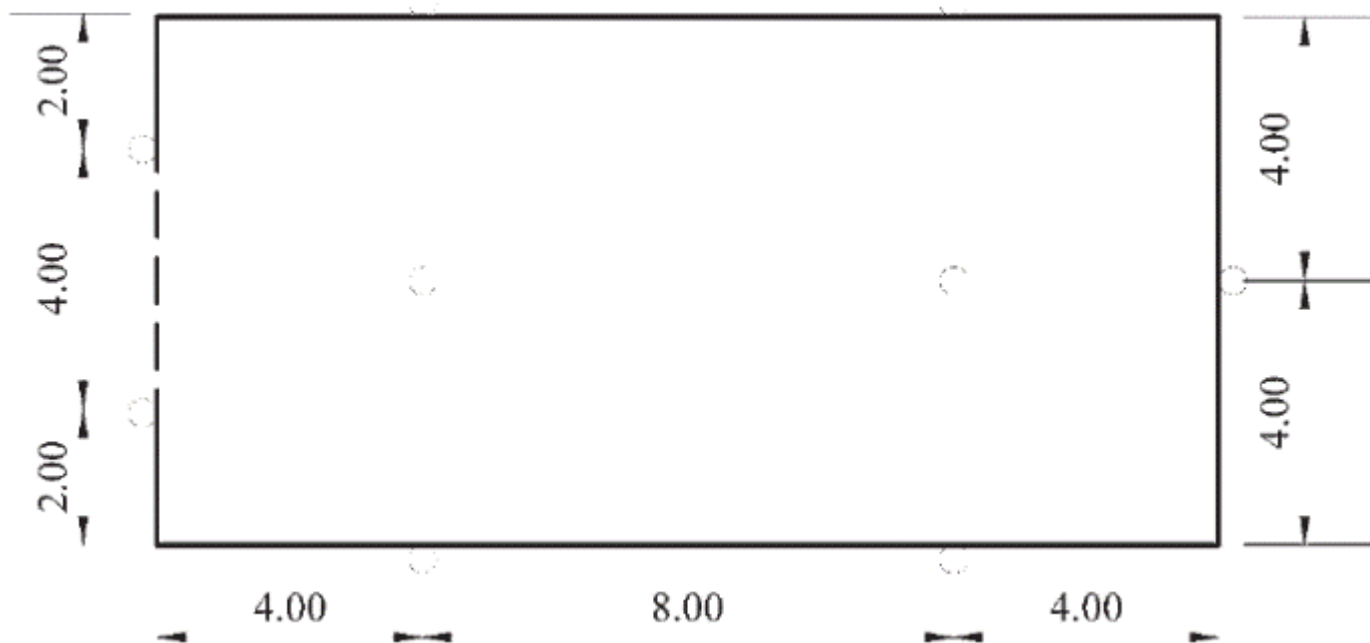
Slika 3. Prostor i oznake prostora za izvođenje poligonske radnje "vožnja putanjom u obliku broja 8" (za osposobljavanje kandidata za vozače motornih vozila kategorija AM, A1, A2 i A)
