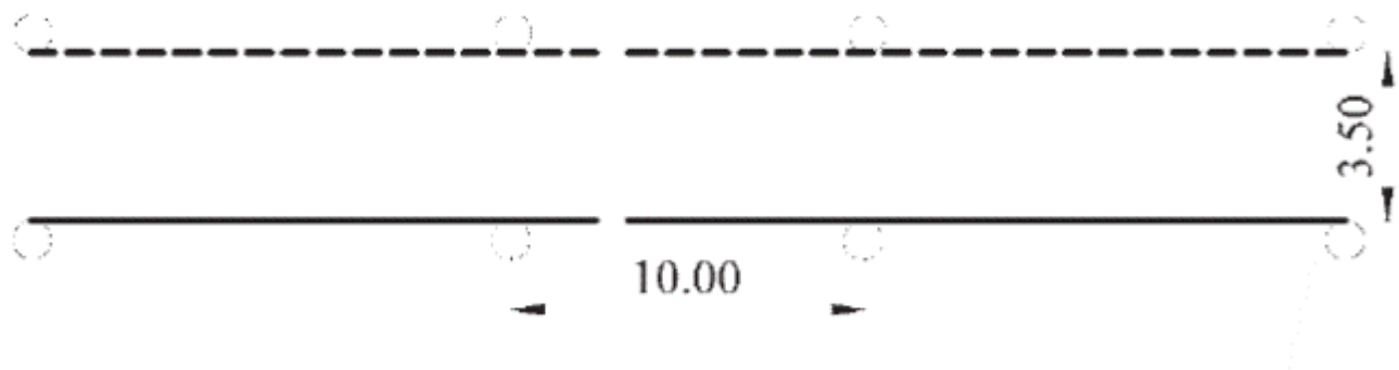
Slika 27. Prostor i oznake prostora za izvođenje poligonske radnje "vožnja napred sa promenom stepena prenosa i unazad u istoj saobraćajnoj traci" (za osposobljavanje kandidata za vozače vozila kategorije M)
