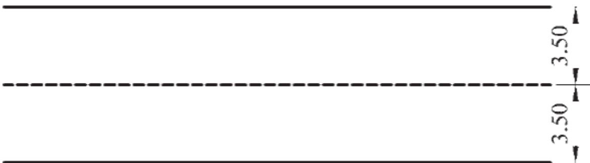
Slika 20. Prostor i oznake prostora za izvođenje poligonske radnje "zaustavljanje vozila na autobuskom stajalištu, radi izlaska i ulaska putnika i polazak sa autobuskog stajališta" (za osposobljavanje kandidata za vozače vozila kategorija D1 i D)
