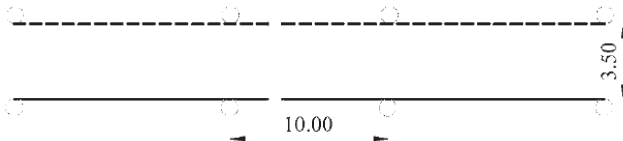
Slika 16. Prostor i oznake prostora za izvođenje poligonske radnje "odvajanje i spajanje vučnog i priključnog vozila" (za osposobljavanje kandidata za vozače vozila kategorija C1E i CE)
