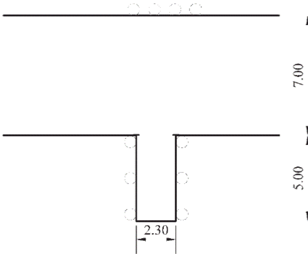
Slika 7. Prostor i oznake prostora za izvođenje poligonske radnje "parkiranje vozila pod pravim uglom, vožnjom unazad" (za osposobljavanje kandidata za vozače motornih vozila kategorija B1 i B)
