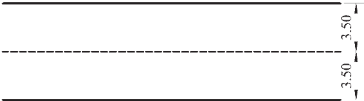
Slika 24. Prostor i oznake prostora za izvođenje poligonske radnje "odvajanje i spajanje vučnog i priključnog vozila" (za osposobljavanje kandidata za vozače vozila kategorije F)
